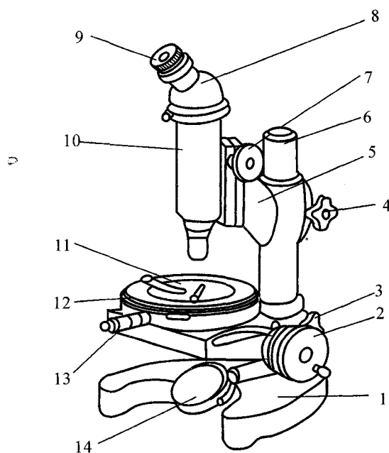
图4 测量显微镜外形图
