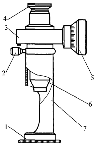
图3 读数显微镜外形图之三
